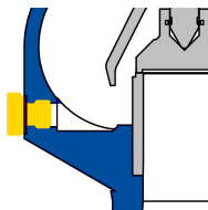
Ausführung mit Ablassschraube
