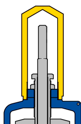
Hebellose Ausführung
