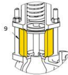
Ausführung mit Zwischenaufsatz 610, 630
