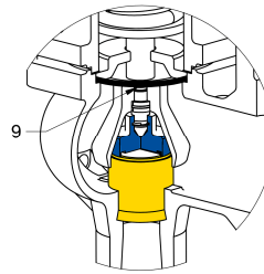
630 Ausführung: 01 Abdichtung -4
