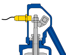
Ausführung mit induktivem Sensor
