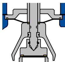
Mit Membran Ausführung (01-4)
