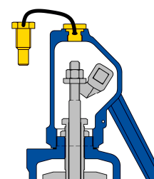
Ausführung mit Feststellschraube (test gag)
