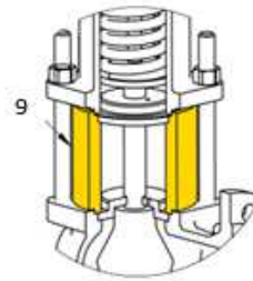
Ausführung mit Zwischenaufsatz 613, 673
