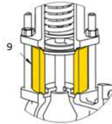
Ausführung mit Zwischenaufsatz 610, 630
