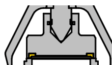
Ausführung mit Weichsiegel (-2, -3)
