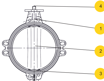
Ausführung 497 DN500 - DN700
