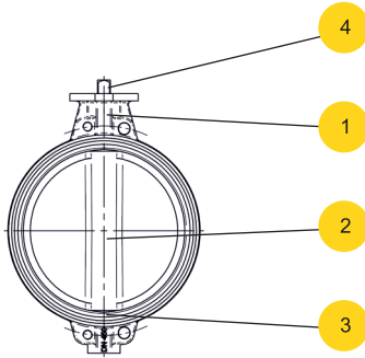
Ausführung 497 DN450
