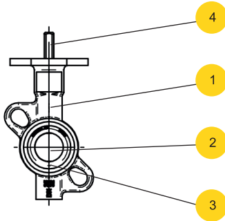
Ausführung 497 DN450
