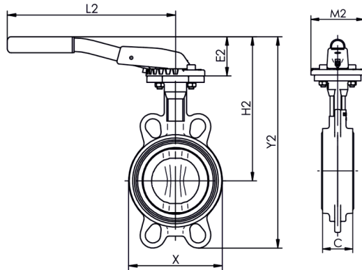
Hebel 497 DN32 - DN200
