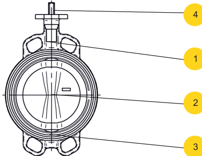
Ausführung 497 DN40 - D400
