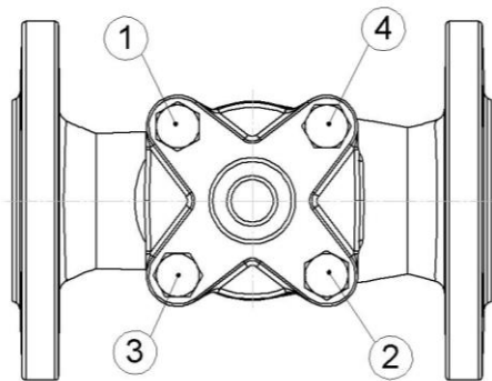
Reihenfolge, in der die Schrauben zur Verbindung des Gehäuses mit dem Deckel festzuziehen sind
